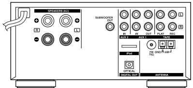
CR-H228i CD-Receiver mit Eingang für iPod Docking-Station
