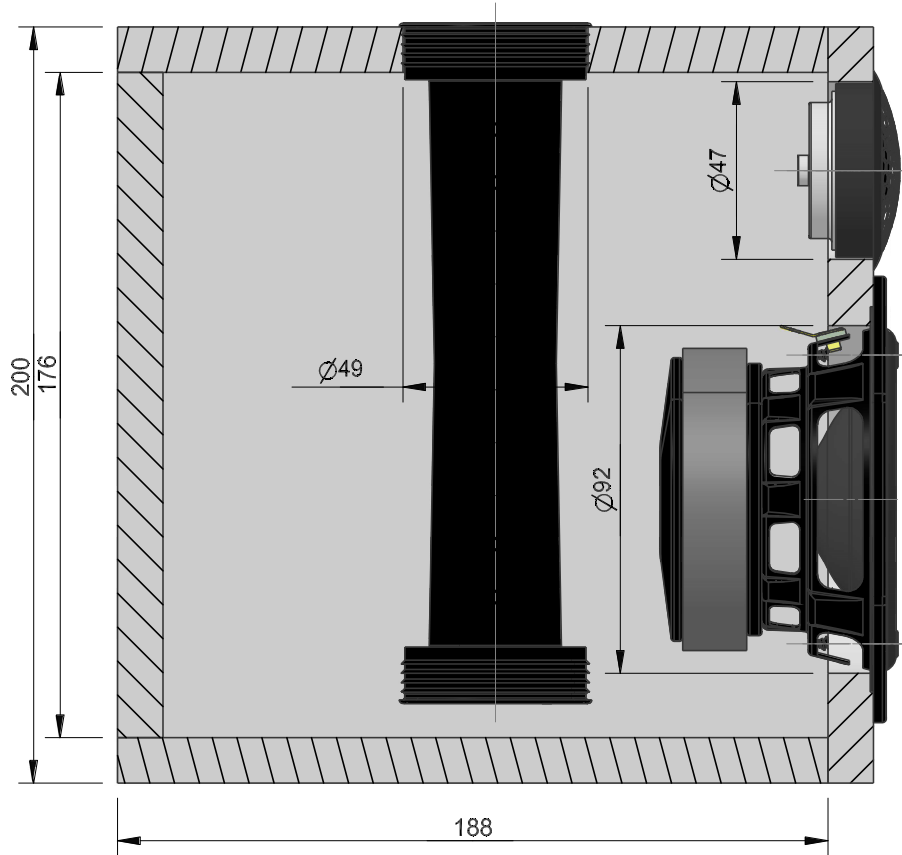
Schnitt A-A
